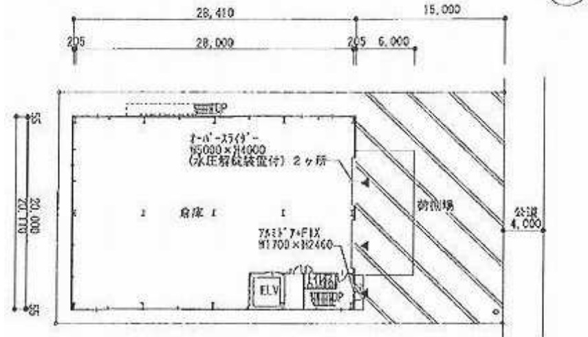
配置・1階平面図
