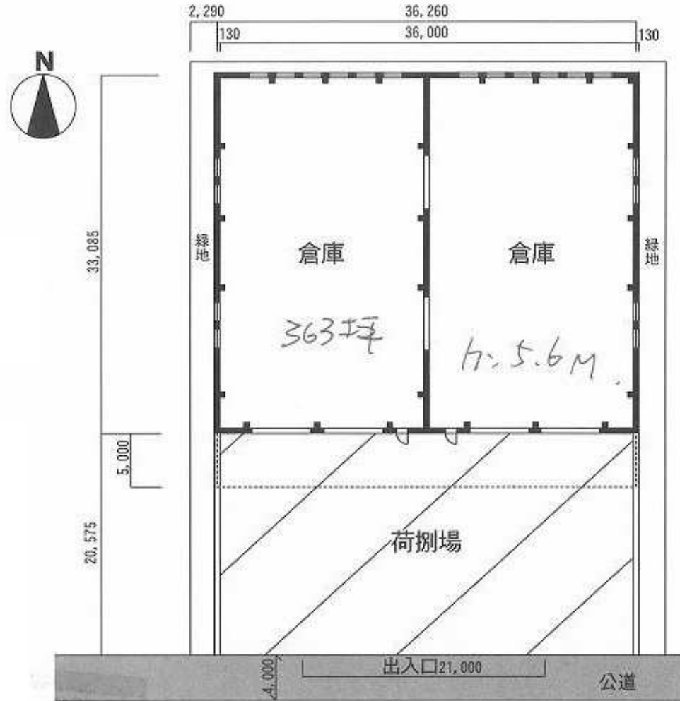
【配置・平面図】
